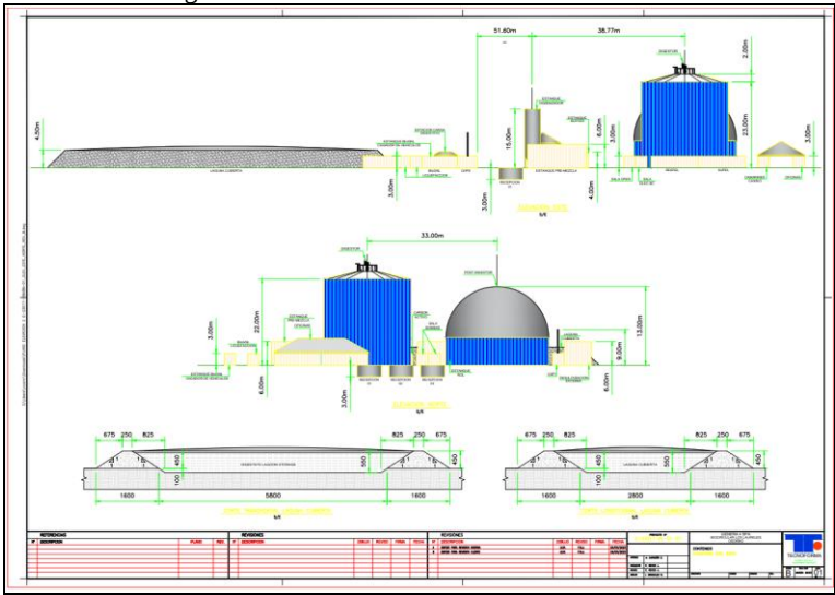
Figura 10: Plano de elevaciones lado Este-Norte.
