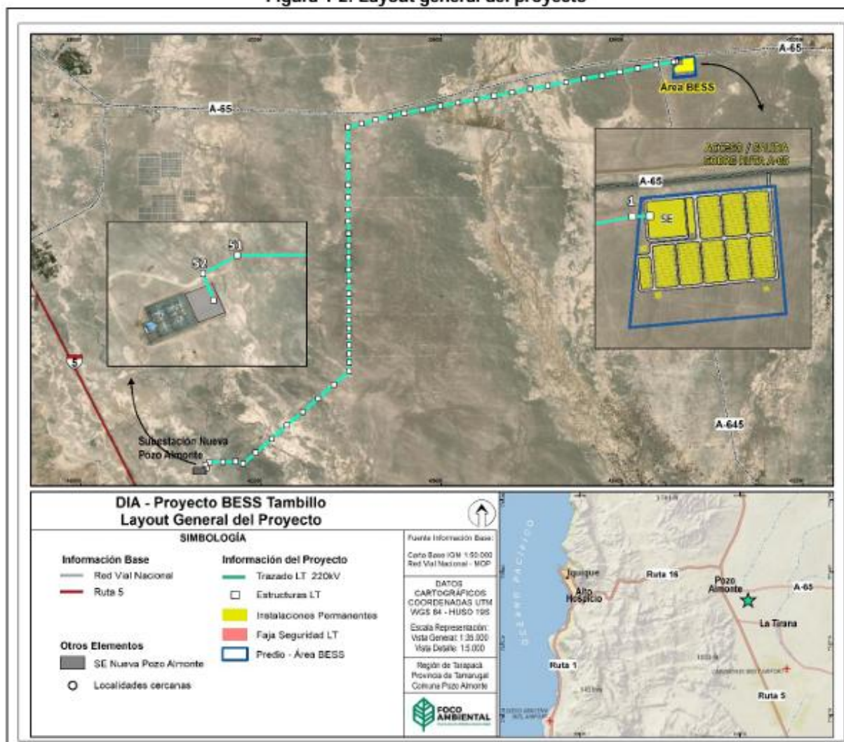
Figura 1-2: Layout general del proyecto
