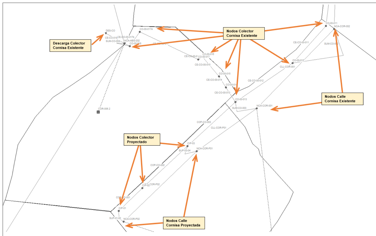
Figura 5-4 Implementación del Colector Projectado y Calle Projectada en Modelación SWMM.
