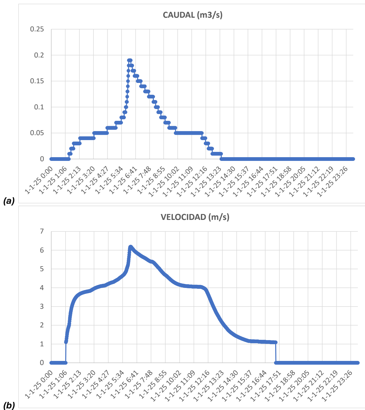
Figura 4-4 Caudal (a) y velocidad (b) versus tiempo, en Colector Cornisa, tramo CE-CO-00-016. Tormenta T=2 años y D=12 horas.
