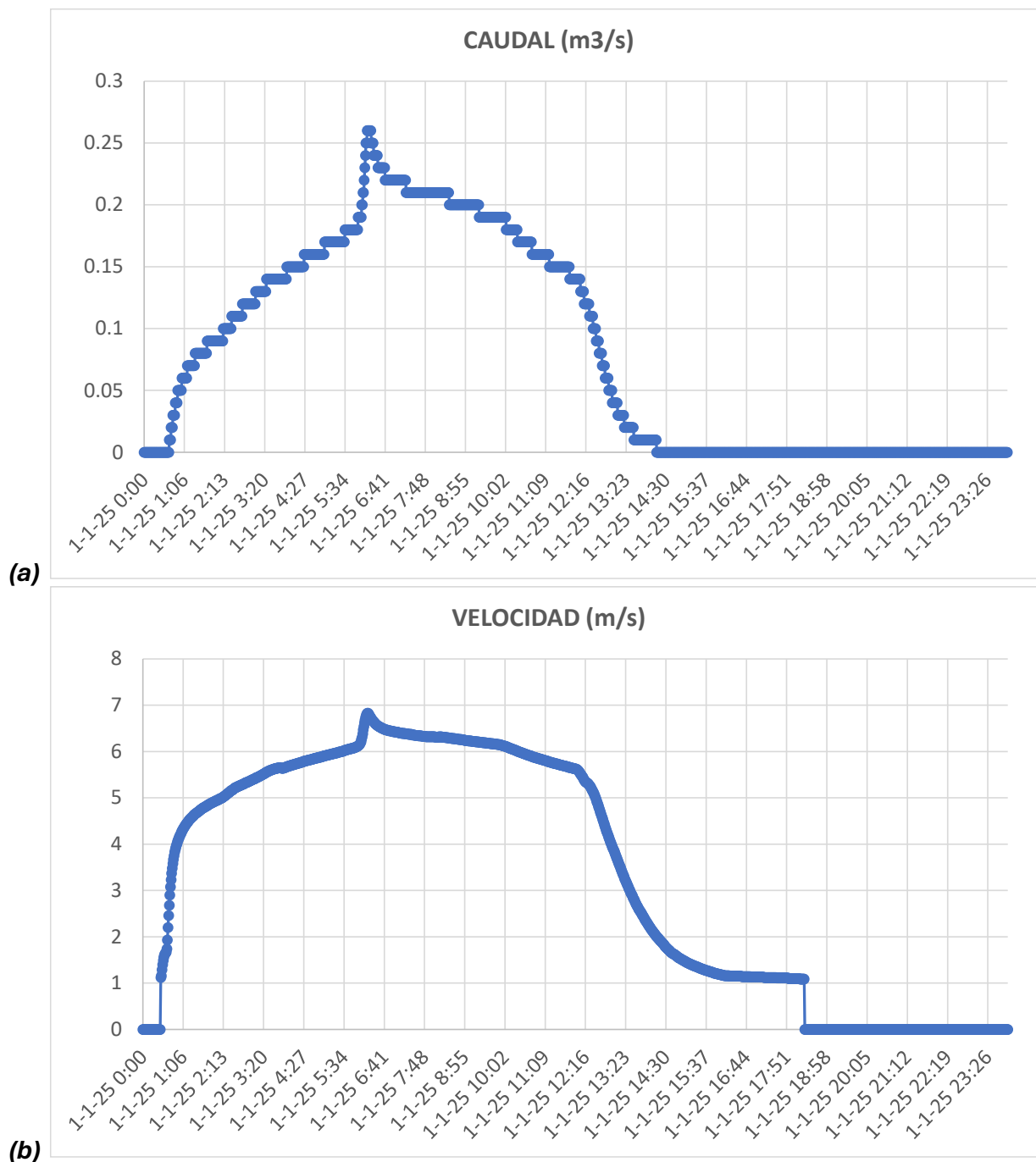
Figura 6-3 Caudal (a) y velocidad (b) versus tiempo, en Colector Cornisa, tramo CE-CO-00-016. Tormenta CP-SCC_T100D12
