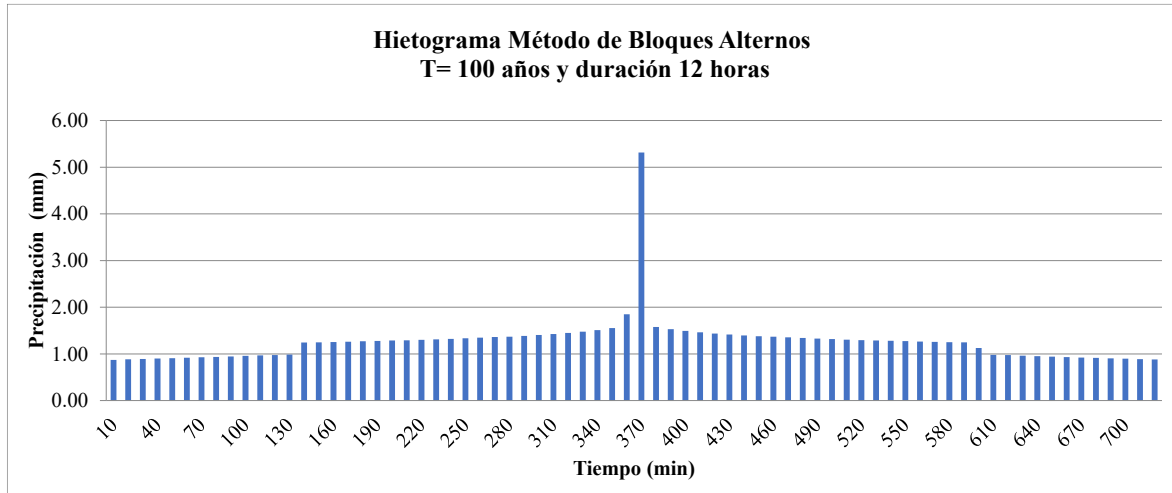
Figura 5-2 Hietograma de la Tormenta Escenario Con Cambio Climático, T100 D12, Precipitación : 91,09 mm.
