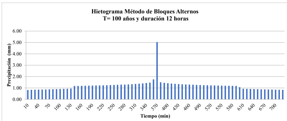
Figura 5-1 Hietograma de la Tormenta Escenario Sin Cambio Climático, T100 D12, Precipitación : 86,28 mm.
