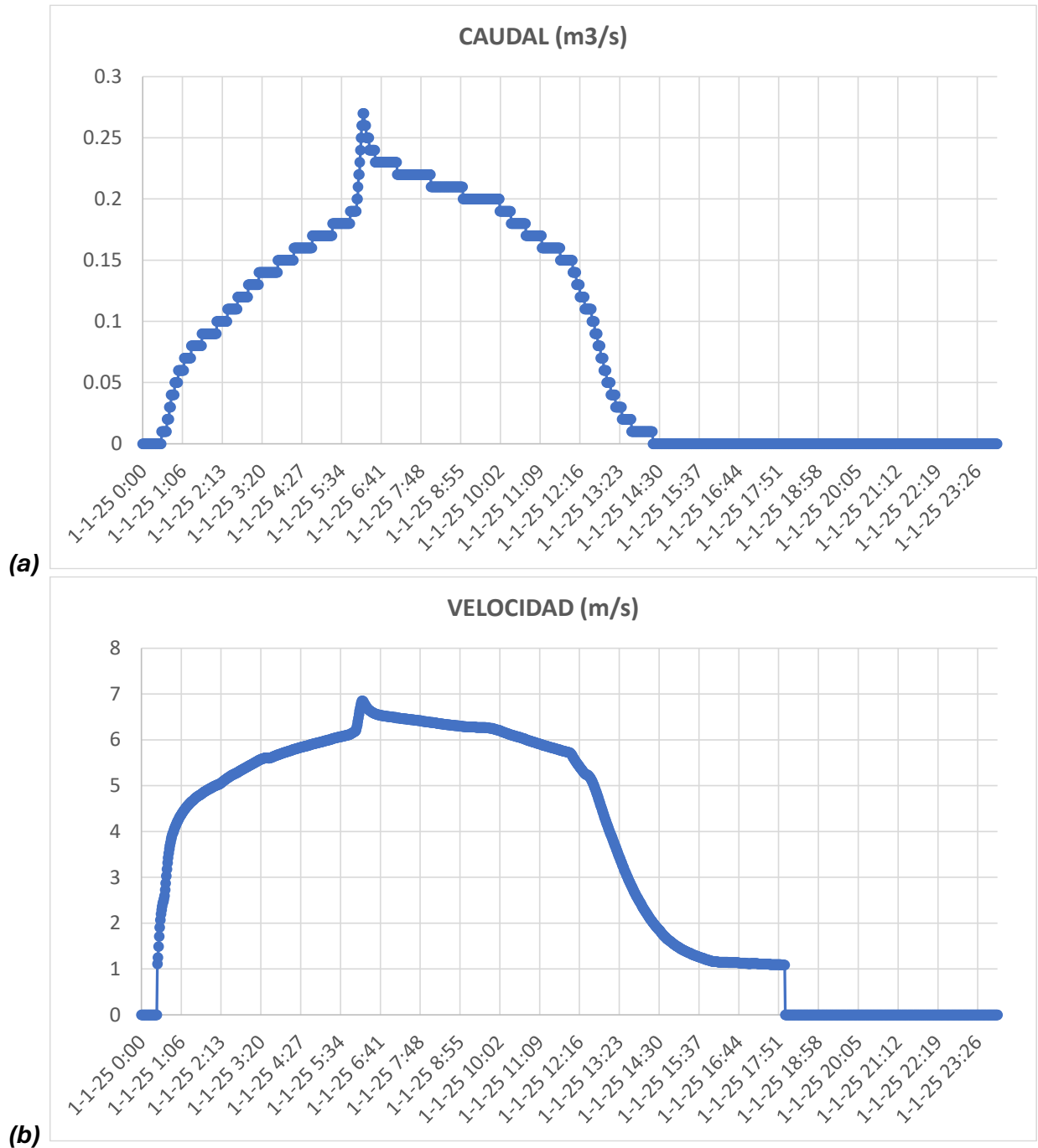
Figura 6-2 Caudal (a) y velocidad (b) versus tiempo, en Colector Cornisa, tramo CE-CO-00-016. Tormenta SP-CCC_T100D12
