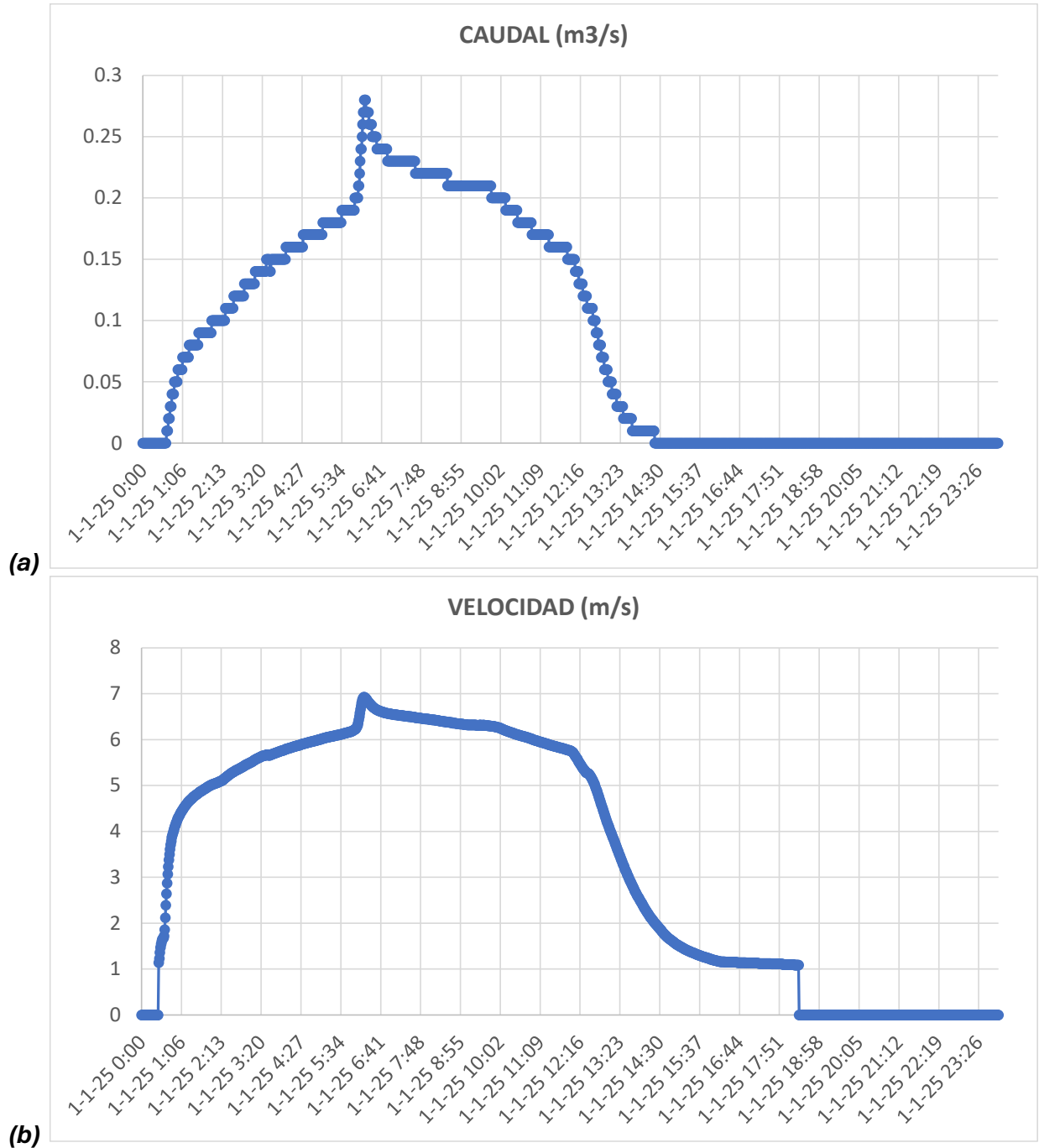
Figura 6-4 Caudal (a) y velocidad (b) versus tiempo, en Colector Cornisa, tramo CE-CO-00-016. Tormenta CP-CCC_T100D12.
