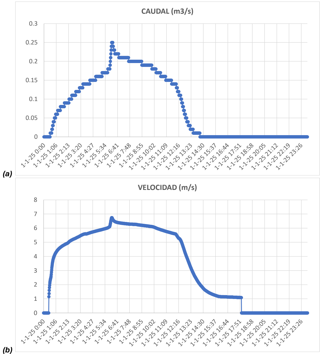
Figura 6-1 Caudal (a) y velocidad (b) versus tiempo, en Colector Cornisa, tramo CE-CO-00-016. Tormenta SP-SCC_T100D12
