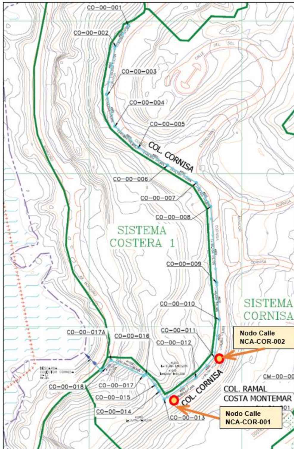
Figura 4-5 Colector Cornisa y Cámaras de Inspección.
